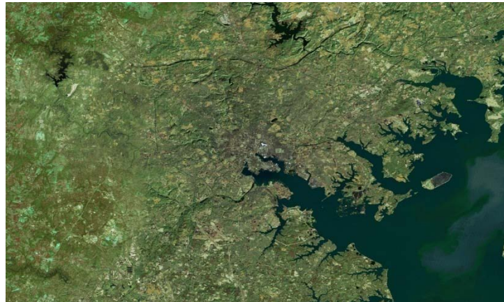
MODIS
